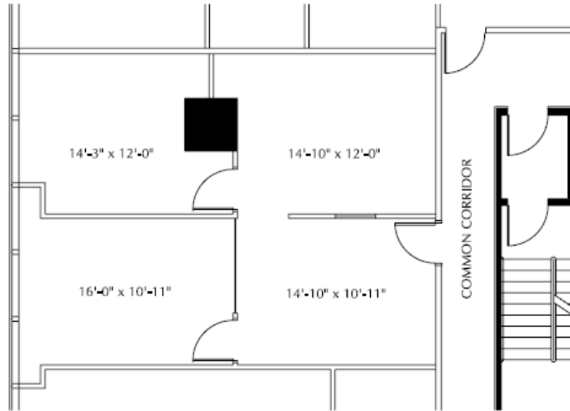
FLOOR PLAN N.T.S.
